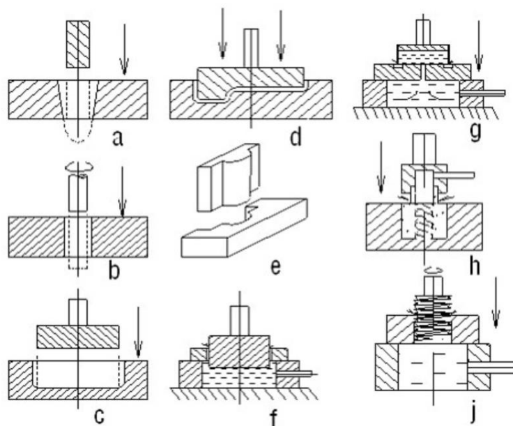
Một số phương pháp gia công bằng tia lửa điện
