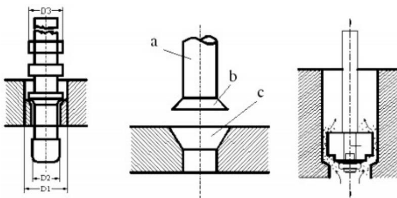
Một số đầu điện cực côn
