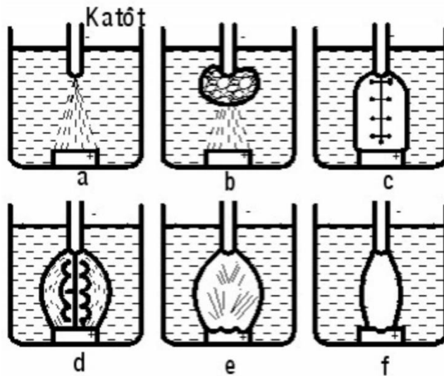
Quá trình hình thành sự phóng tia lửa điện
